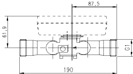
Całkowita długość 190 mm (przyłącze gwintowe)
